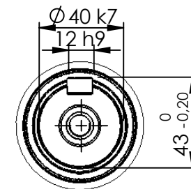
DETTAGLIO A
